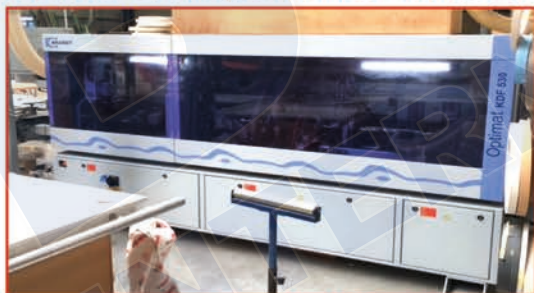
Plaqueuse de chant OPTIMAT KDF 530
